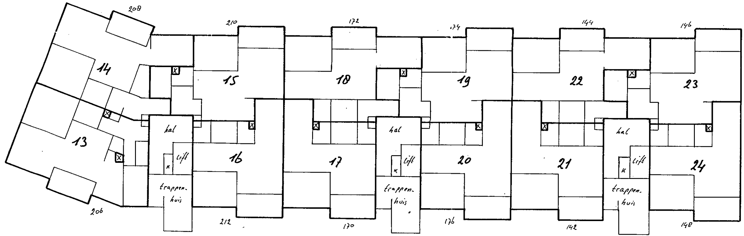
1e VERDIEPING 1:200
