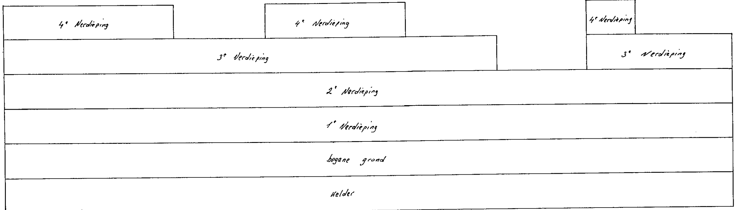
DOORSNED E A-B 1:200
