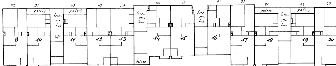
1e VERDIEPING 1:200
