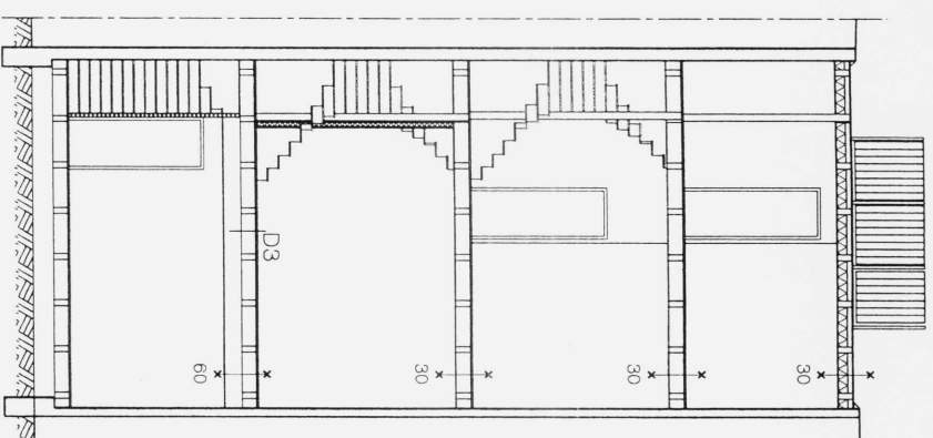
doorsnede A-A
