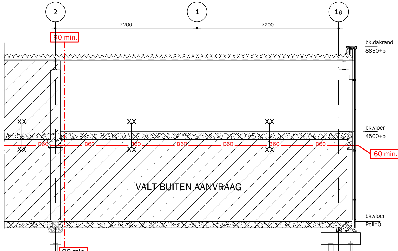
Doorsnede A-A - bestaande toestand
