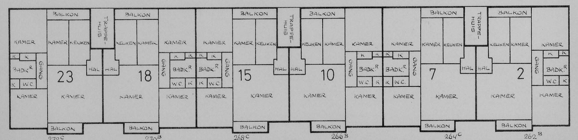
1e étage 1 : 200
