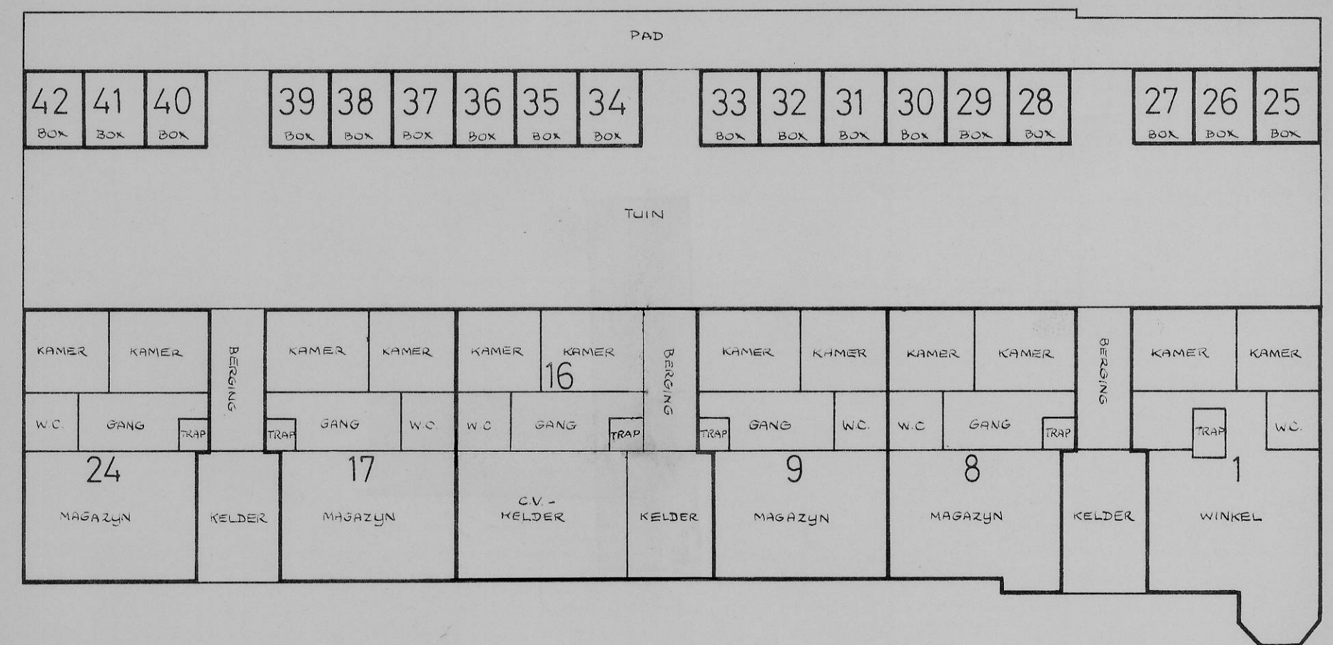
sousterrain 1 : 200
