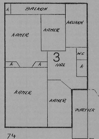
2e Verdieping 1:200
