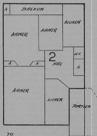
1e Verdieping 1:200
