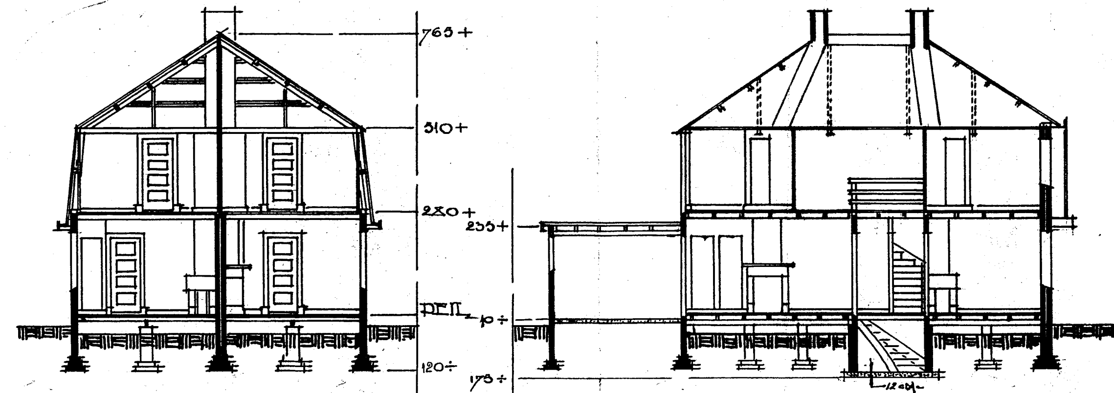
• DOORSNEDE ~ A •
