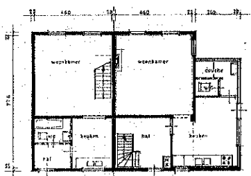
begane grond
