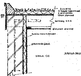
balklaag verdiepingvloer
