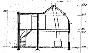
doorsnede a-a
