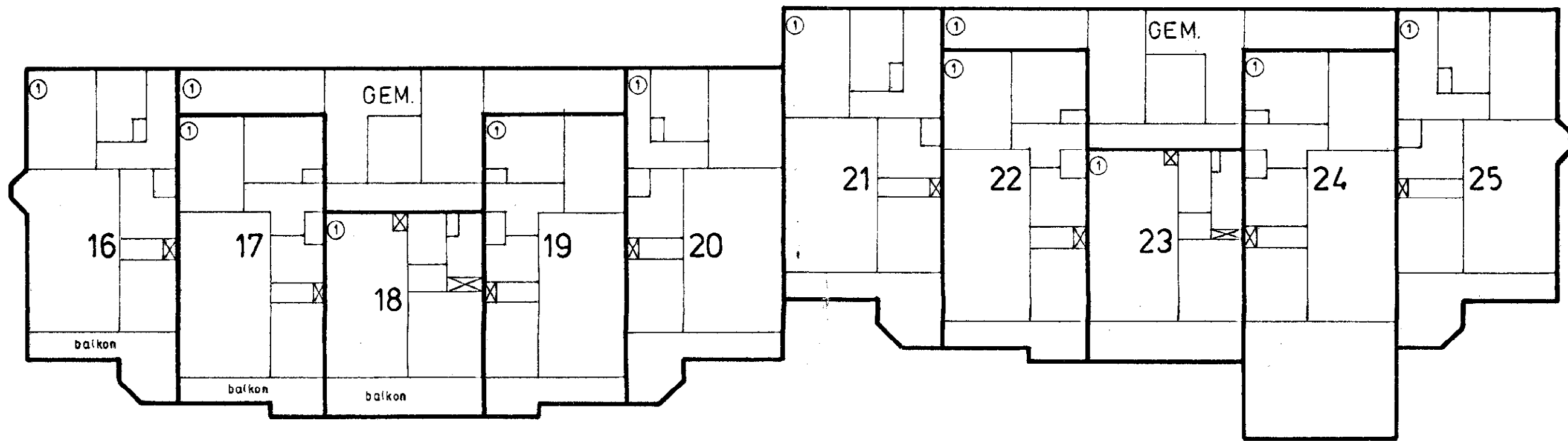
1e verdieping
