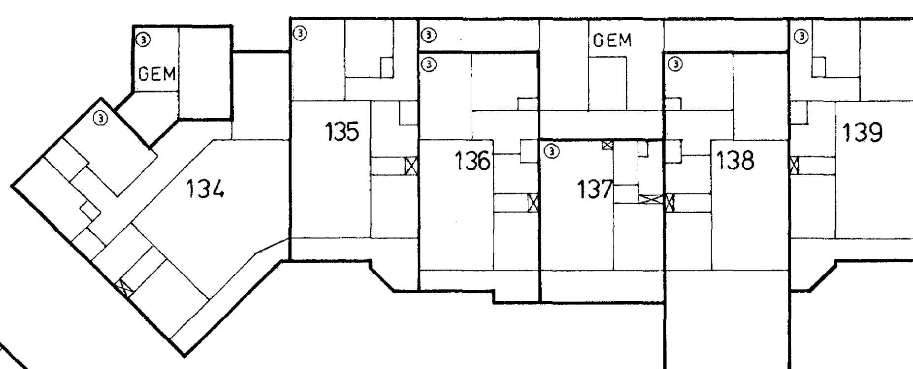
3e verdieping
