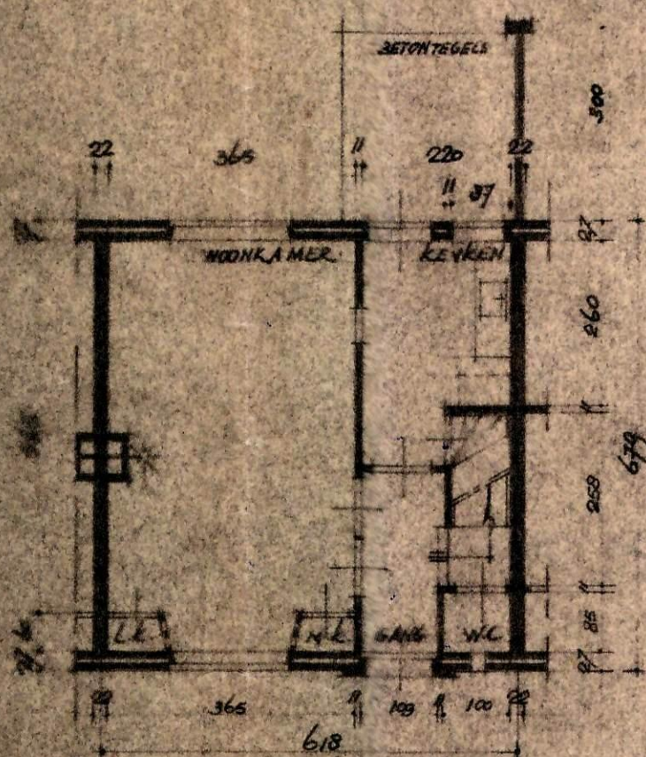
BEGANE GROND
