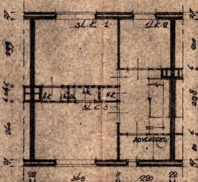
VERDIEPING
