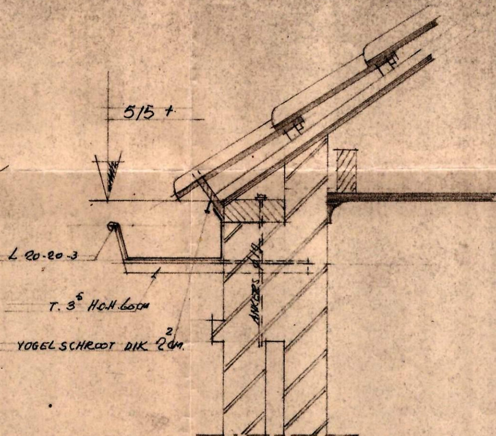
DAKVOET TYPE I
