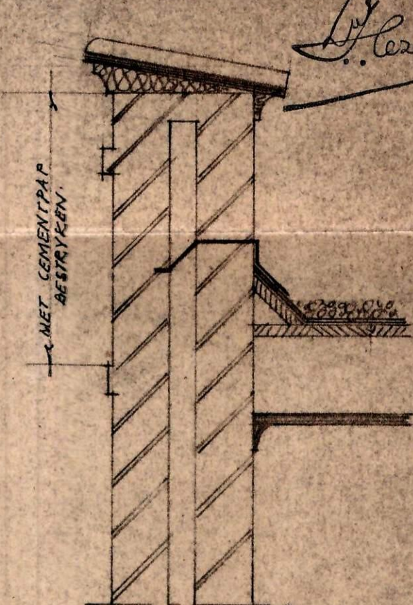
GEVEL BEEIND AANBOUWEN
