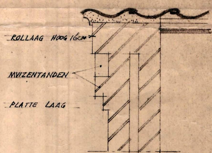
GEVEL BEEINDIGING
