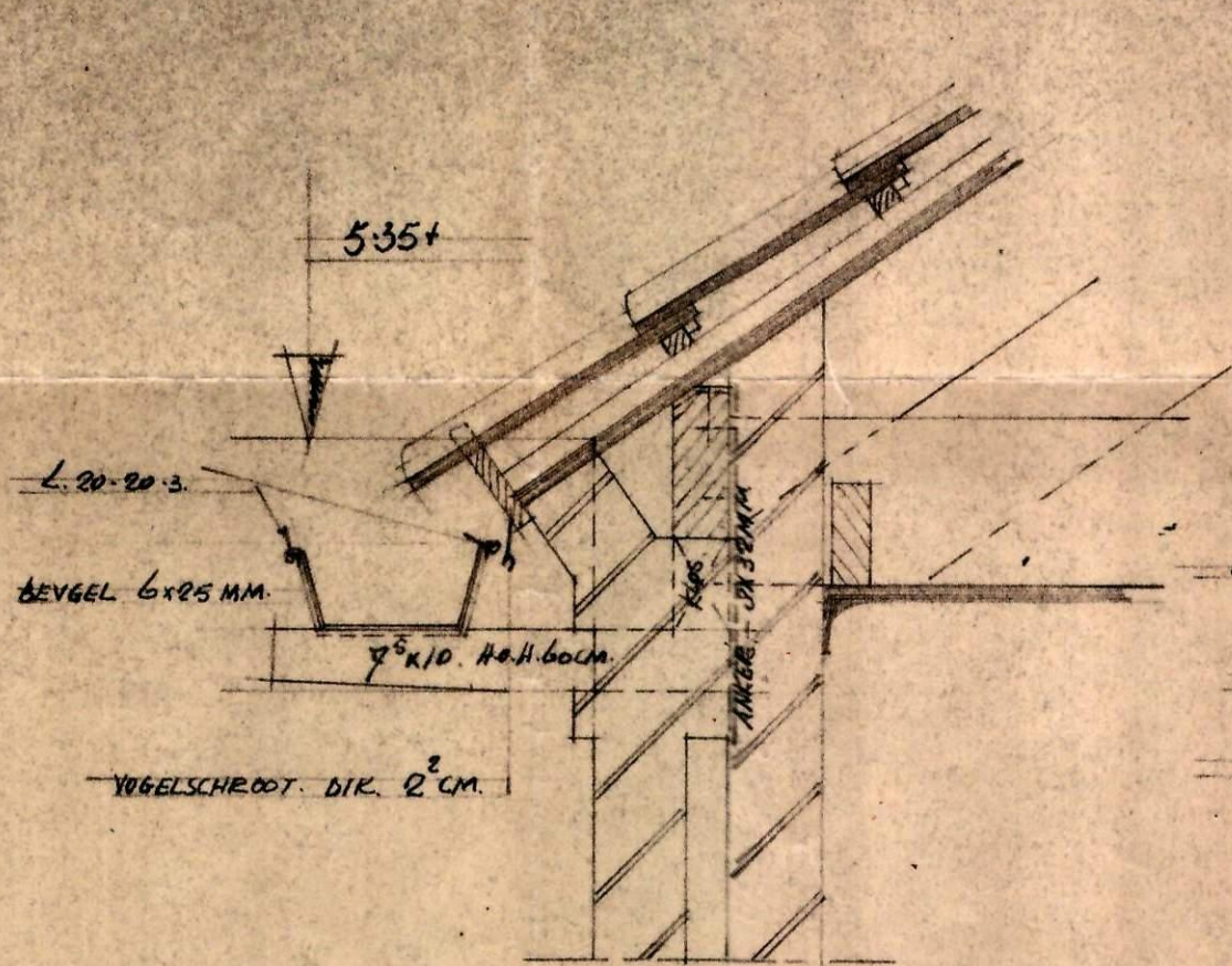
DAKVOET TYPE II
