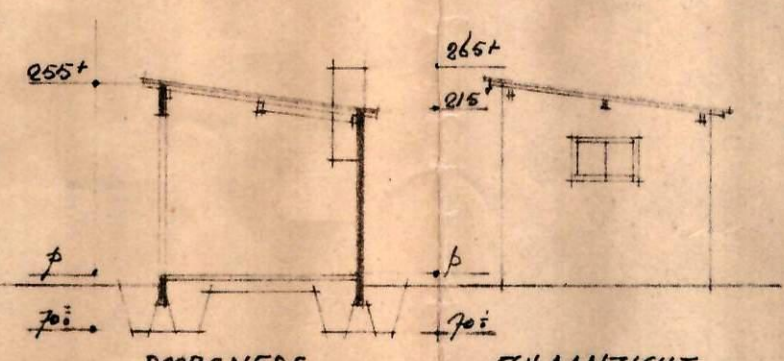
DOORSNEDE
