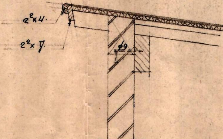
DET A BERGING
