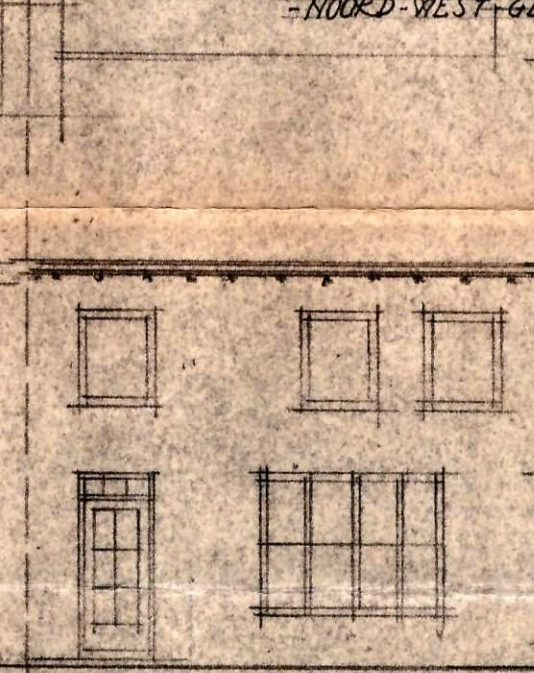
ACHTERGEVEL
