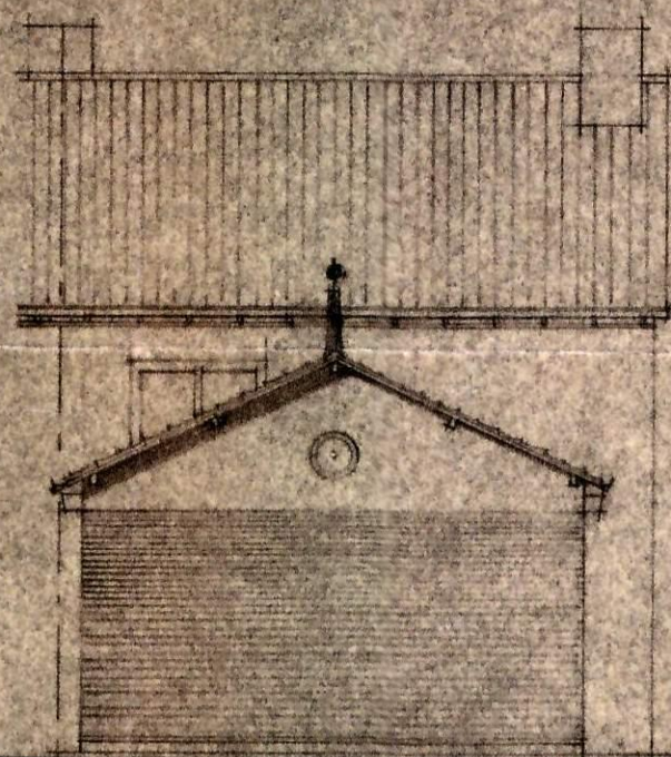
ZUID-WEST-GEVEL
