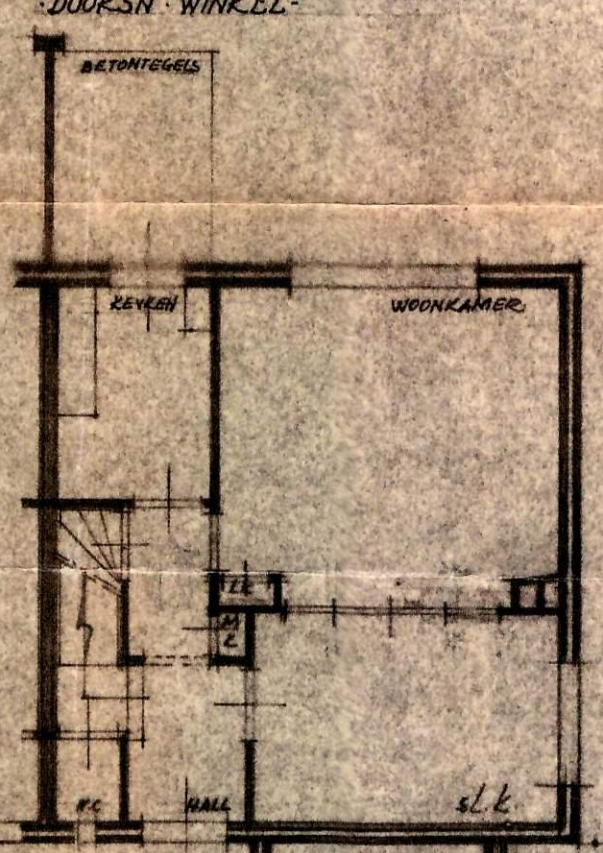
DOORSN. WINKEL
