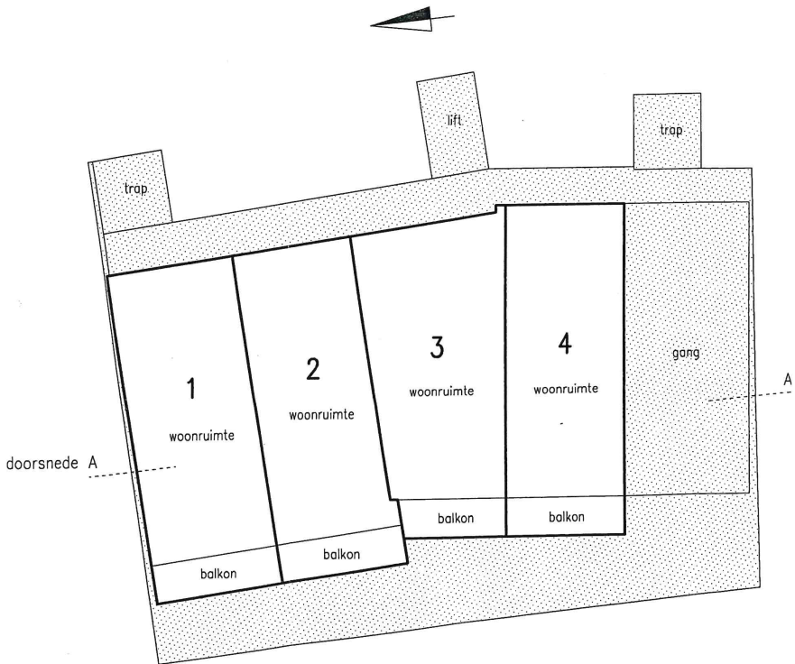
BEGANE GROND schaal 1 : 200
