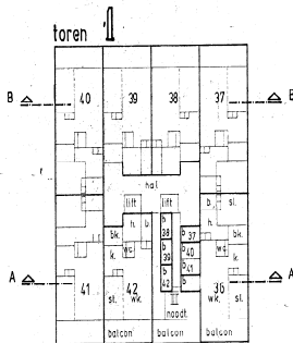
5e Verdieping 1:200
