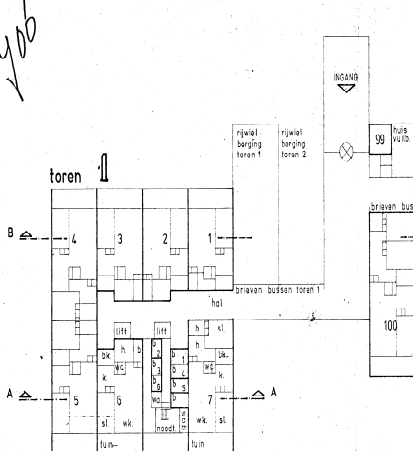
11e Verdieping 1: 200
