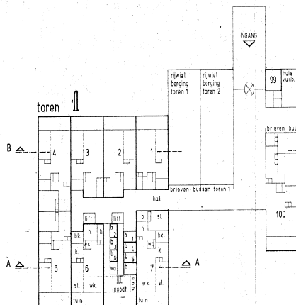
2e V verdieping 1:200
