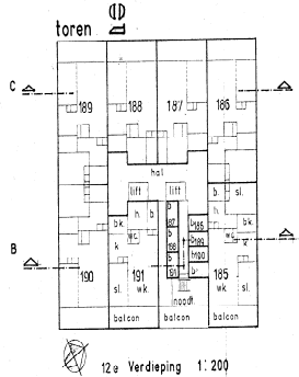
12e Verdieping 1: 200
