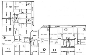
2e VERDIEPING 1:100
