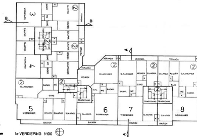
1e VERDIEPING 1:100
